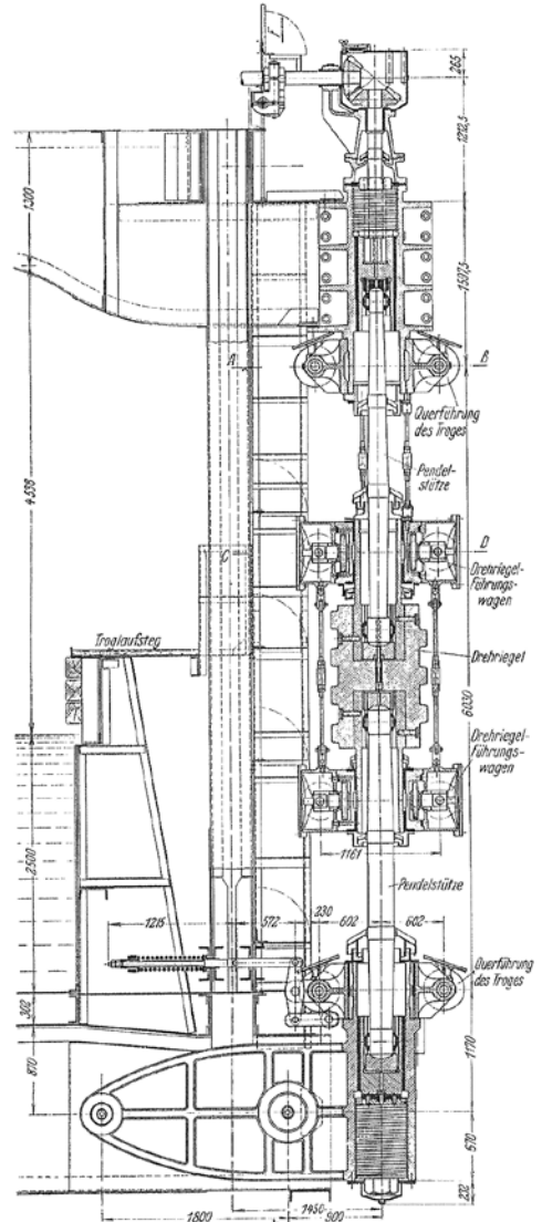
Drehriegel
