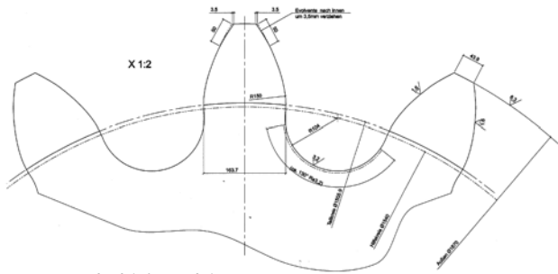
Lantaarn rondsel (uitsnede)
