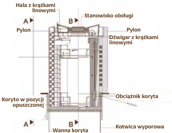
Przekrój
